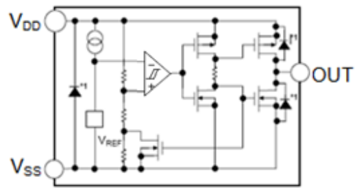
CMOS output
